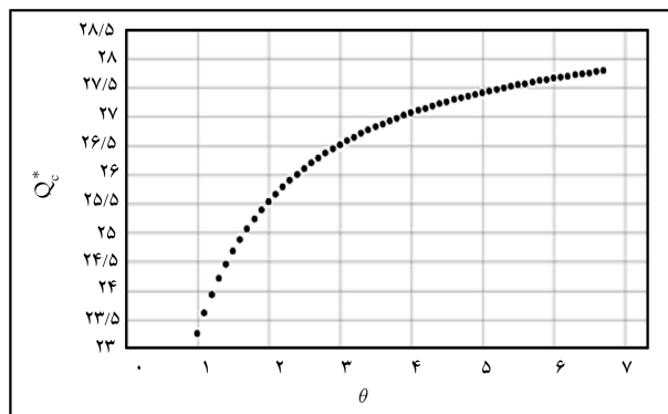
شکل ۱۲. تغییرات اندازه‌ی دسته‌ی تولید محصول نهایی بر اساس تغییرات نرخ دوباره‌کاری قطعات a و b نسبت به تولیدشان.
