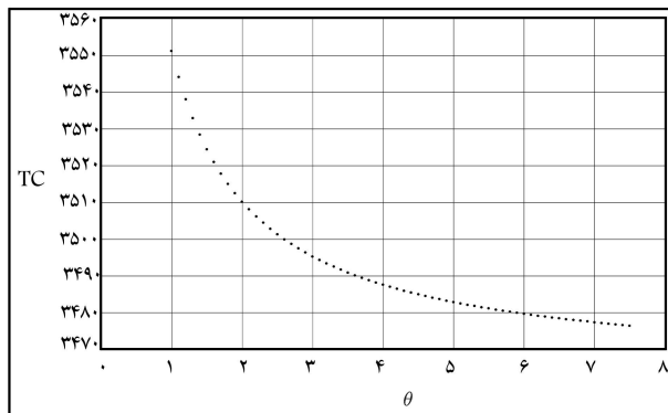
شکل ۱۱. تغییرات هزینه‌ی کل موجودی نسبت به تغییر نرخ دوباره‌کاری قطعات a و b نسبت به نرخ تولیدشان.
