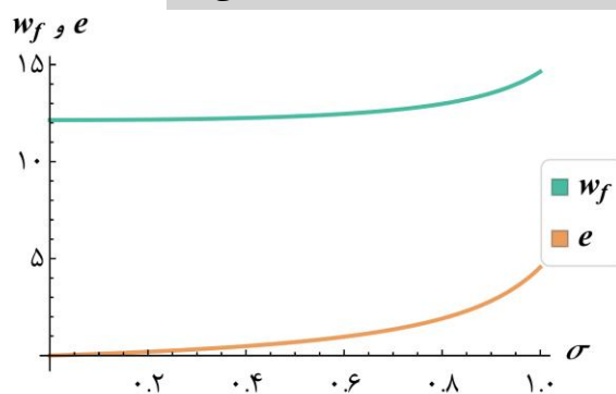
شکل ۱ نمودار مربوط به روند تغییرات w_f و e نسبت به تغییرات \sigma
