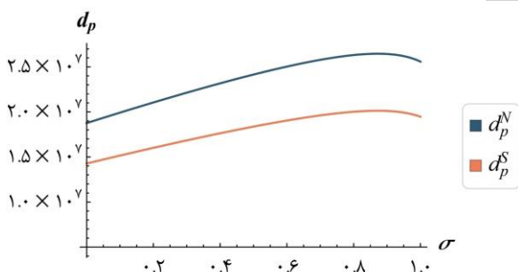
شکل ۳ نمودار مربوط به روند تغییرات تقاضاهای تعادلی تولیدکننده در دو ساختار نش و استکلبرگ نسبت به تغییرات \sigma
