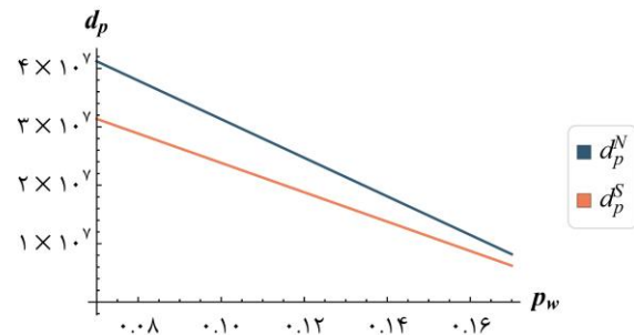
شکل ۱۲ نمودار مربوط به روند تغییرات تقاضاهای تعادلی تولیدکننده در ساختار نش و استکلبرگ نسبت به تغییرات p_w
