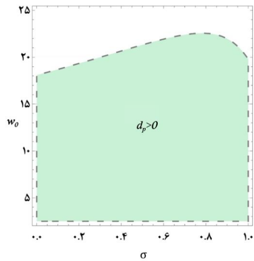
شکل ۵ نمودار مربوط به ناحیه تقاضاهای تعادلی مثبت تولیدکننده در ساختار نش و استکلبرگ نسبت به تغییرات \sigma و w_0
