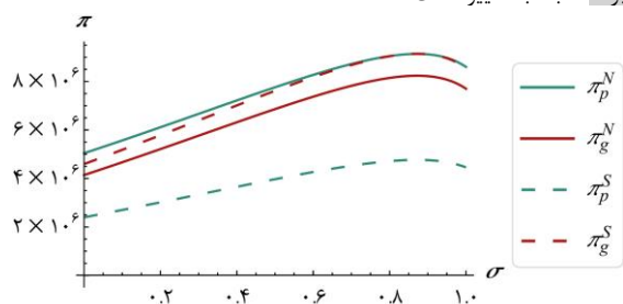
شکل ۴ نمودار مربوط به روند تغییرات سودهای تعادلی دولت و تولیدکننده در ساختار نش و استکلبرگ نسبت به تغییرات \sigma
