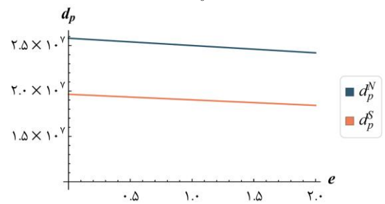
شکل ۶ نمودار مربوط به روند تغییرات تقاضاهای تعادلی تولیدکننده در ساختار نش و استکلبرگ نسبت به تغییرات e
