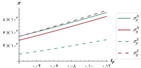
شکل ۱۰ نمودار مربوط به روند تغییرات سودهای تعادلی دولت و تولیدکننده در ساختار نش و استکلبرگ نسبت به تغییرات t_p
