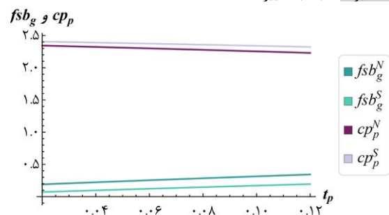
شکل ۸ نمودار مربوط به روند تغییرات سوبسید پرداختی دولت به مصرف‌کننده و قیمت نهایی مصرف‌کننده در حالت تعادل در ساختار نش و استکلبرگ نسبت به تغییرات t_p
