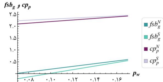
شکل ۱۱ نمودار مربوط به روند تغییرات سوبسید پرداختی دولت به مصرف‌کننده و قیمت نهایی مصرف‌کننده در حالت تعادل در ساختار نش و استکلبرگ نسبت به تغییرات p_w
