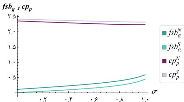
شکل ۲ نمودار مربوط به روند تغییرات سوبسید پرداختی دولت به مصرف کننده و قیمت نهائی مصرف کننده در حالت تعادل در دو بازی نش و استکلبرگ نسبت به تغییرات \sigma
