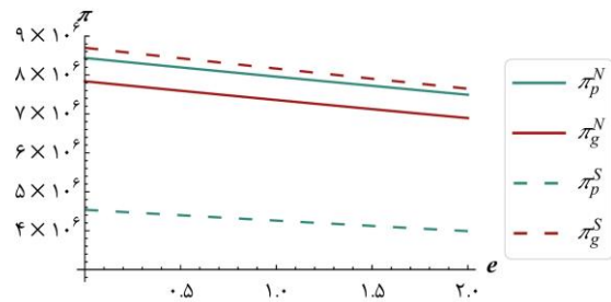
شکل ۷ نمودار مربوط به روند تغییرات سودهای تعادلی دولت و تولیدکننده در دو ساختار نش و استکلبرگ نسبت به تغییرات e
