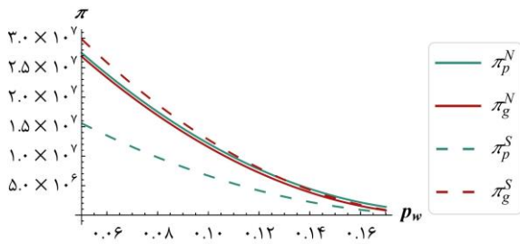
شکل ۱۳ نمودار مربوط به روند تغییرات سودهای تعادلی دولت و تولیدکننده در ساختار نش و استکلبرگ نسبت به تغییرات p_w
